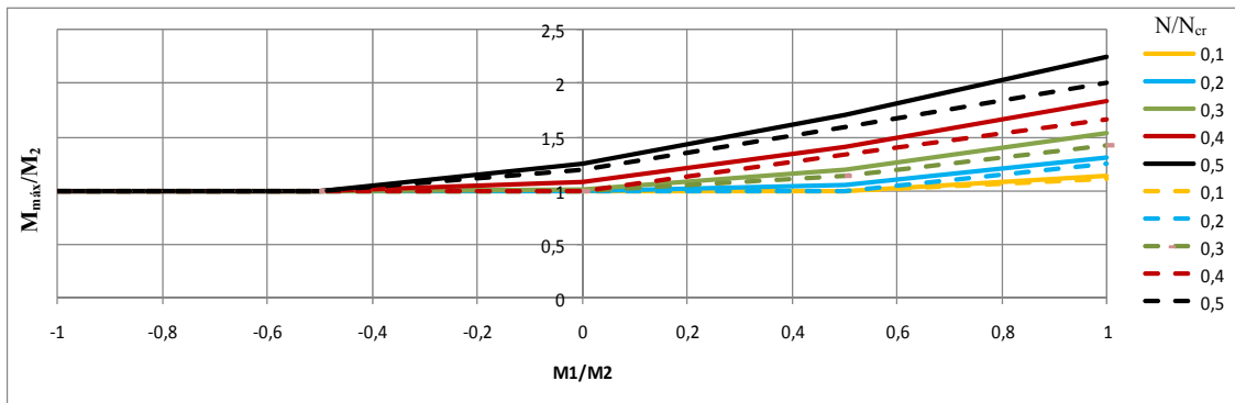
Figura 4.8 – Valores de M_{\text{máx}}/M_2 exatos (linha cheia) e aproximados (linha tracejada) \geq 1
