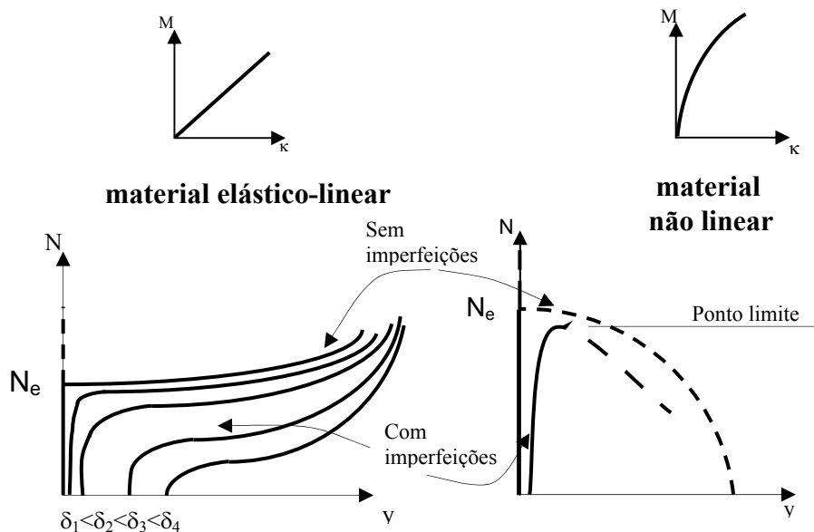
Figura 2.14 - Gráfico N x y de pilares com imperfeições geométricas
