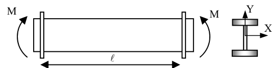
Figura 3.18 - Flexão pura. Seção I
