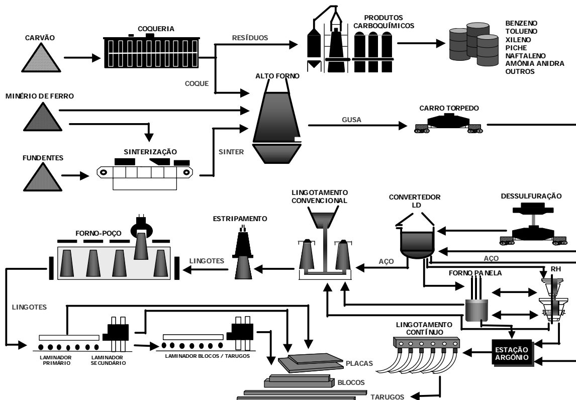
Figura 1.1 – Fluxo de processo siderúrgico
