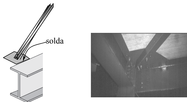
Figura 5.18 - Ligação entre travamento vertical e pilar
