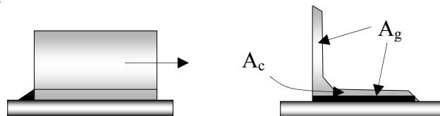
Figura A.3 - Força de tração transmitida somente por soldas transversais
