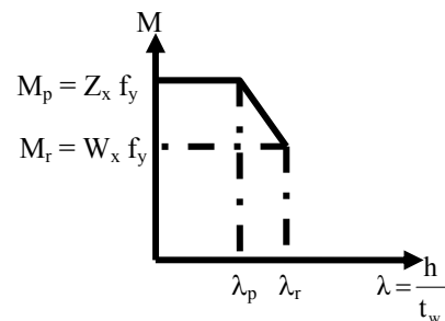
Figura 3.9 Gráfico M_{Rk} x \lambda na instabilidade local de alma
