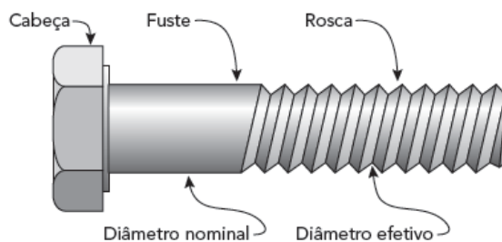
Figura 5.1- Parafuso.
