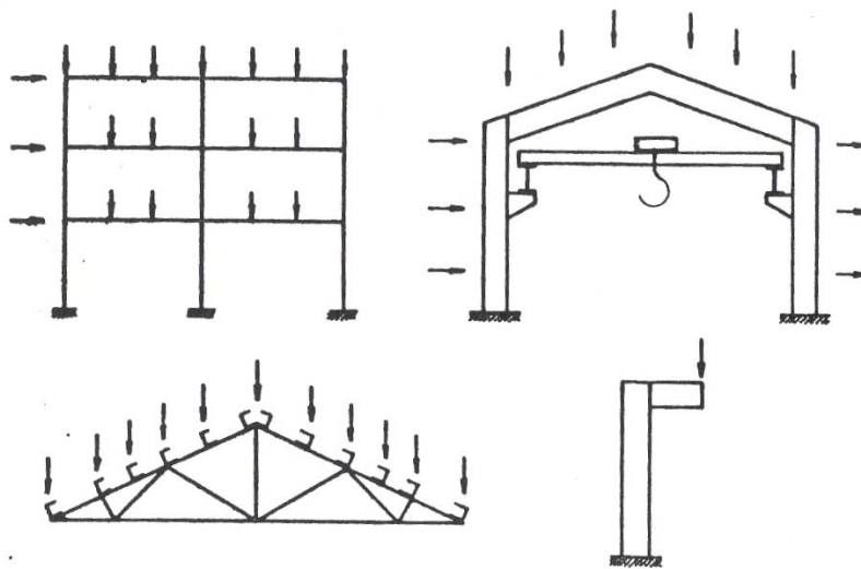
Figura 4.1 – Exemplos de peças sob flexão composta.
