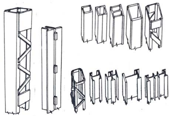
Figura 3.8 - Exemplo de perfis compostos utilizados como pilares
